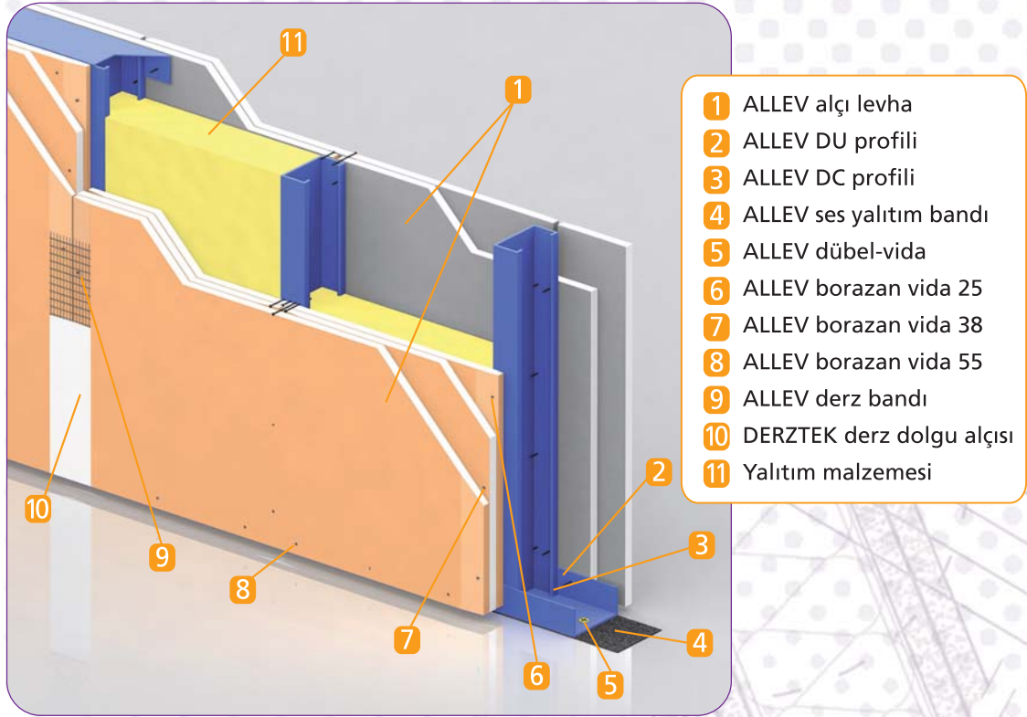
Metal iskeletin bir yüzünde üç kat, diğer yüzünde çift kat alçı levha (3+2) bulunan bölme duvar
